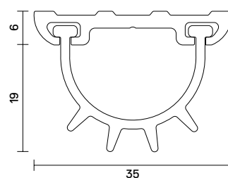
AAS3503 (BLADES OUT) ↑
