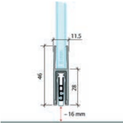
Planet KG-F8
