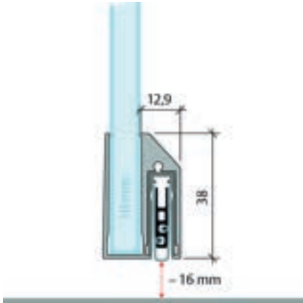
Planet KG-A10
