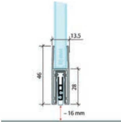
Planet KG-F10
