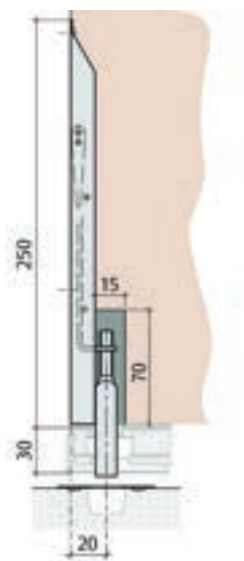
Planet KR Flush Bolt
