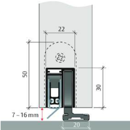
Planet SN
