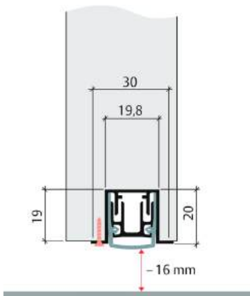
Planet PU
