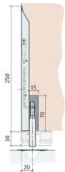
Planet KR Flush Bolt
