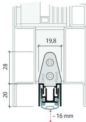
Planet MF PLUS
